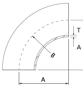
ข้อโค้งสั้นสแตนเลส 90 องศา, 1.5D, 304 และ 316L
