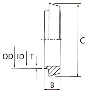
ซีลยูเนียน ,DIN , ทำด้วย SILICONE , EPDM , VITON
