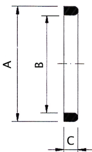
ซีลยูเนียน ,DIN , ทำด้วย SILICONE , EPDM , VITON
